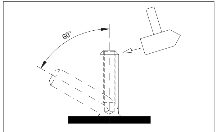
Abb. 12 Prüfung der Schweiss-Stelle nach EN ISO 14 555 (Schlagbiegeversuch) Ill. 12 Vérification de la soudure selon EN ISO 14555 (essai de flexion au choc)
