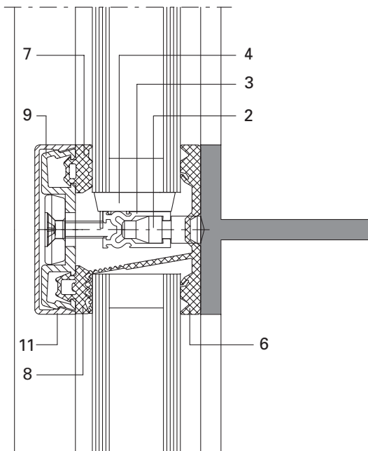
Schweis-Traganker/Boulon-support à souder
