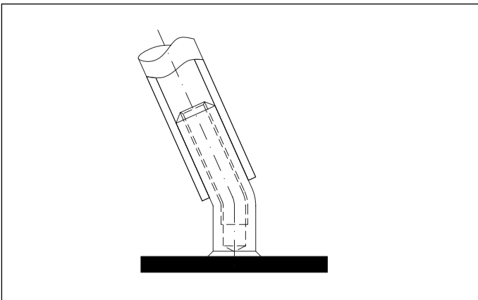
Abb. 11 Prüfung der Schweiss-Stelle nach EN ISO 14555 (Biegeversuch) Ill. 11 Vérification de la soudure selon EN ISO 14555 (essai de flexion)
