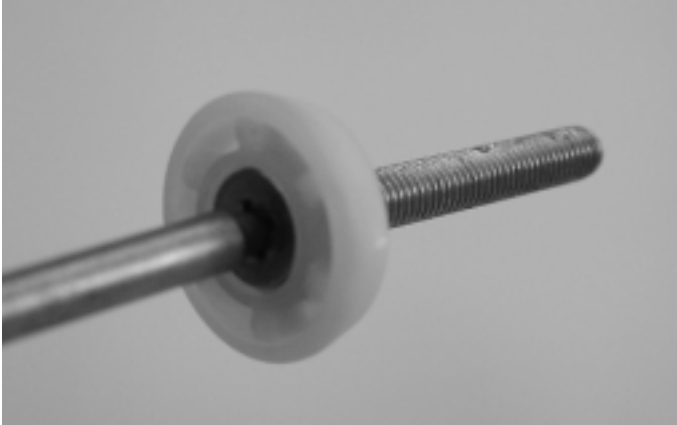
Abb. 27 Spezialschraube M 5 mit Zentrierscheibe auf Schraubklinge SR1 aufgesteckt
