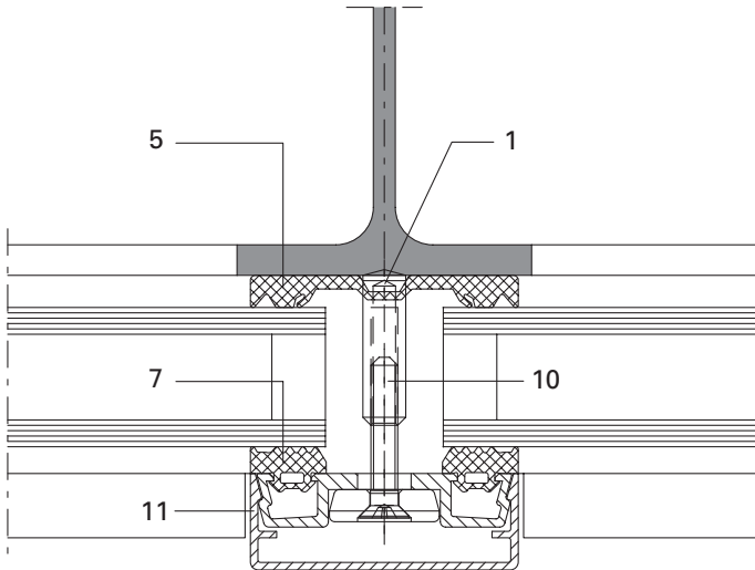
Schweisbolzen/Goujon à souder
